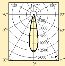
Křivky svítivosti
