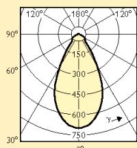
Křivky svítivosti
