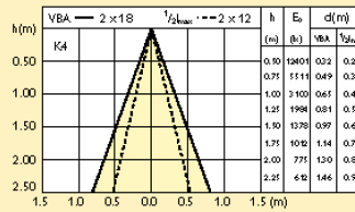
Vyzařovací diagram
