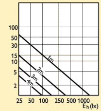
Diagram vizuálního efektu
