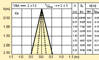
Vyzařovací diagram
