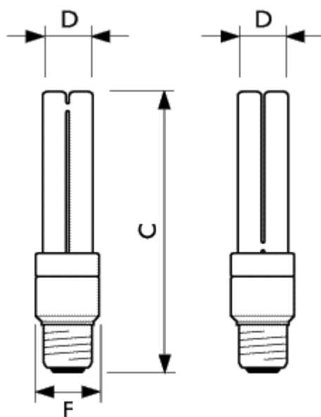
MASTER PL- E E27
