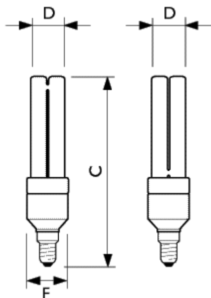
MASTER PL- E E14
