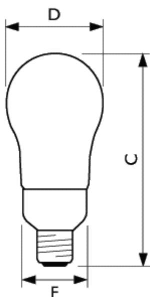
PL- E Ambiance E27 A70/A75/A75A
