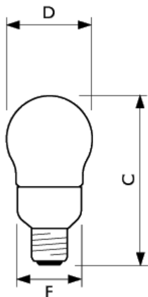
PL- E Ambiance E27 A55/A60C/A65/A65B
