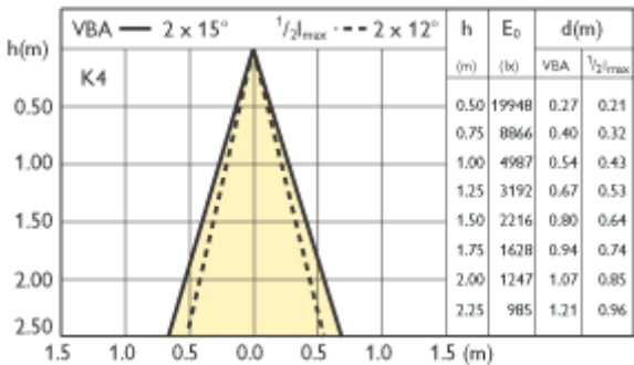
MASTERC CDM-R111 20W 24D
