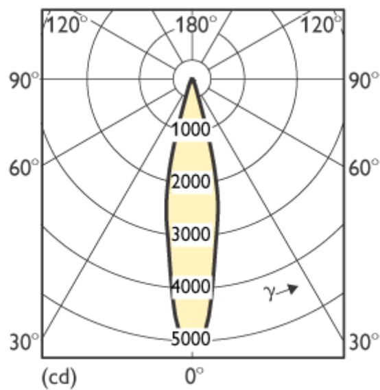
MASTERC CDM-R111 20W 24D
