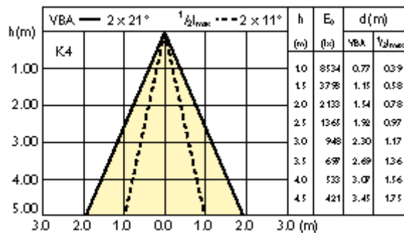
MASTERC CDM-R111 35W 24D
