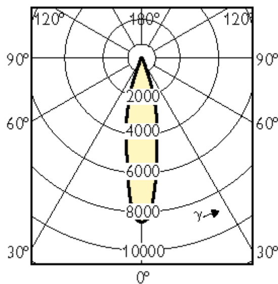
MASTERC CDM-R111 35W 24D
