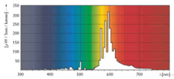
SON 50W/70W
