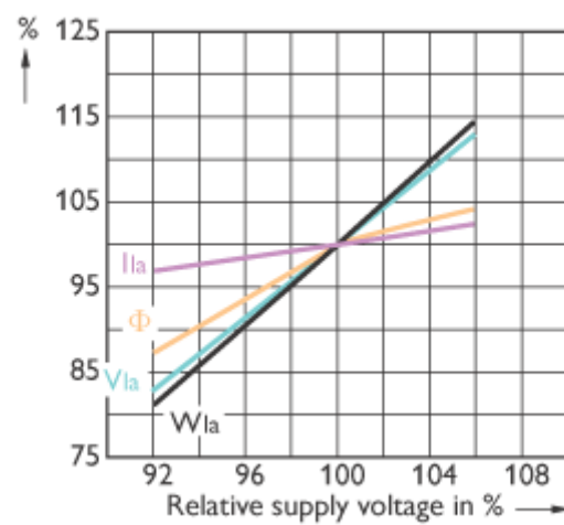
SON 50W/70W
