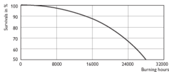
SON 50W/70W
