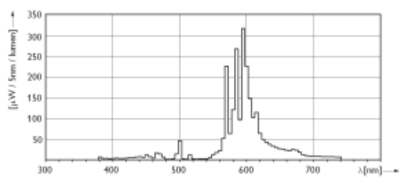
SON 50W/70W
